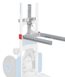
Porte-chaises Capacité de charge 80 kg, nombre max. de chaises env. 15 pièces Art. Nr. 930 183
