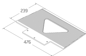
Schaufel GS
