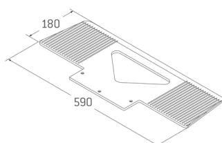
Schaufel XWL
