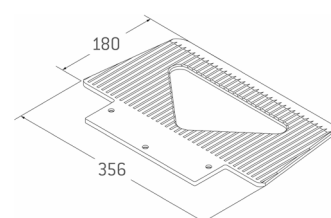
Schaufel WL
